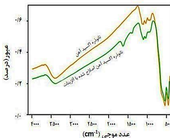
شکل ۷: نمودار نتیجه آزمایش FT-IR مربوط به نانوذره اکسید آهن قبل و پس از اصلاح با آلژینات
