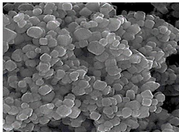
شکل ۱: تصویر حاصل از میکروسکوپ الکترونی نانوذرات اکسید آهن
