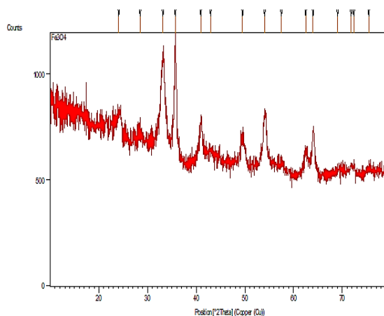
شکل ۶: نتیجه آزمون XRD از نانوذرات اکسید آهن اصلاح شده با آلژینات
