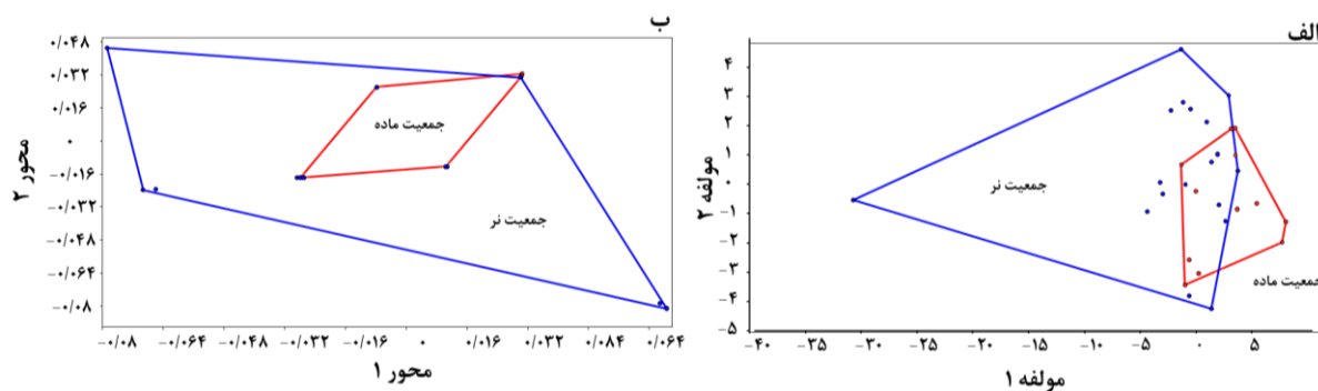
شکل ۲: الف) نمودار پراکنش نمونه‌ها براساس دو مؤلفه اصلی اول صفات اندازه‌ی و ب) رله پلات تجزیه و تحلیل تطابقی (CA relay Plot) صفات شمارشی گاوماهی چشم‌نواری
