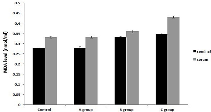
شکل ۱: مقایسه میانگین غلظت MDA در نمونه‌های مایع سمینال و سرم در گروه‌های مختلف
